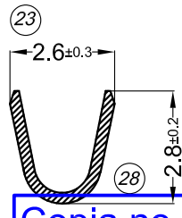
SECC. B-B
